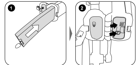
Einschieben des Akkus in die Öffnung des Rahmens
